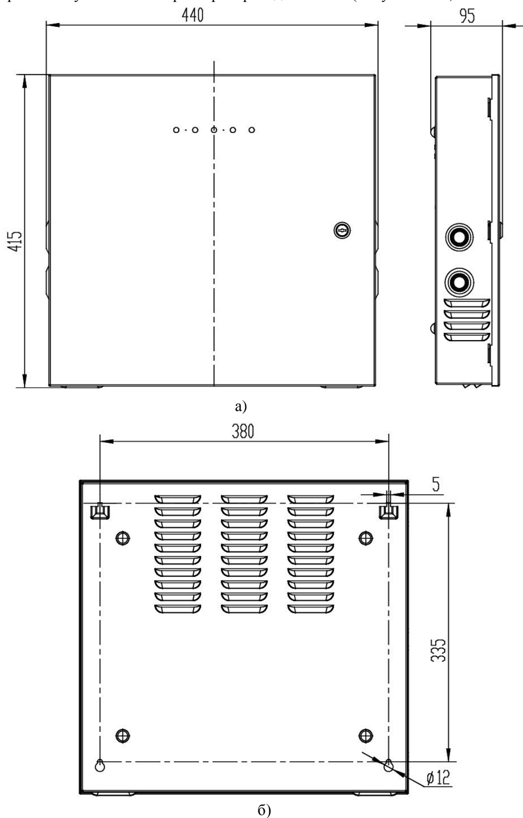
Рисунок 2.2.2. Габаритные и установочные размеры блока.
