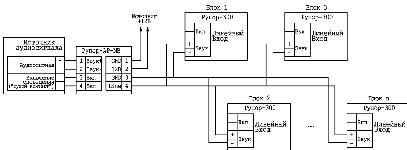
Рисунок 2.2.4. Схема подключения модуля «Рупор-АР-МВ» к блоку «Рупор-300».
