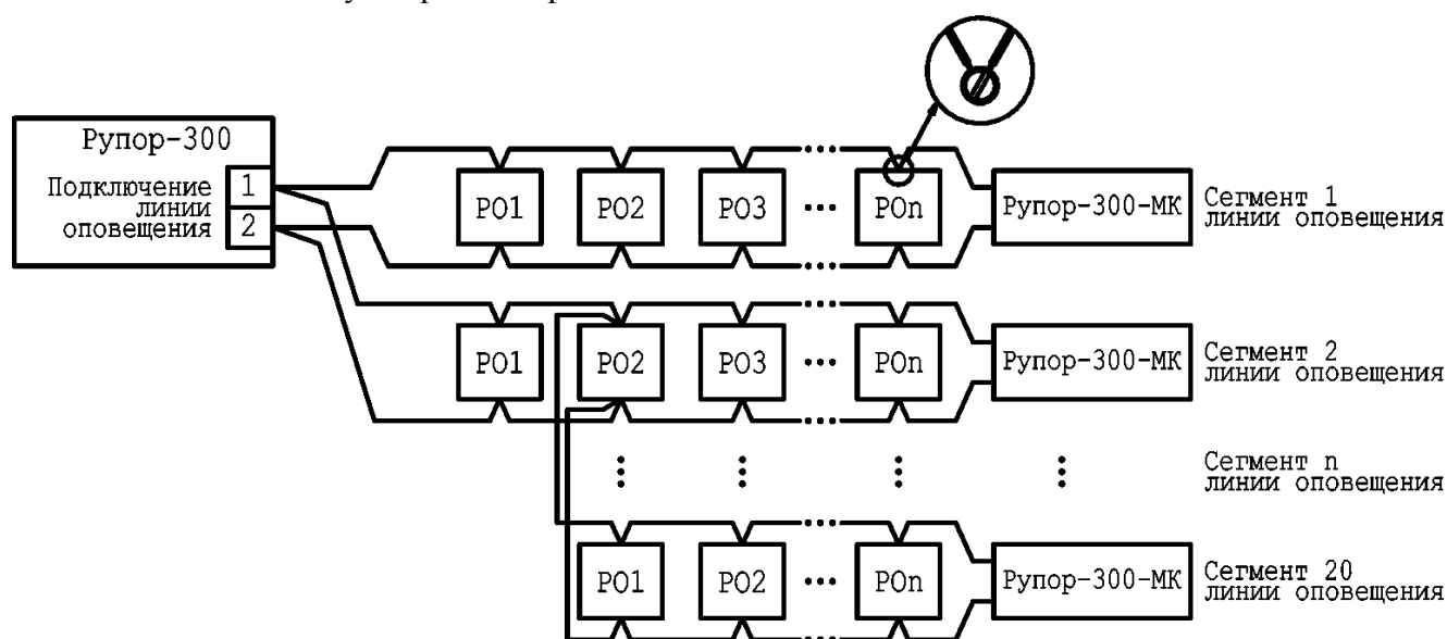
Рисунок 2.2.5. Подключение громкоговорителей к линиям оповещения
