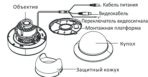
Рисунок 1-1 Внешний вид купольной камеры
