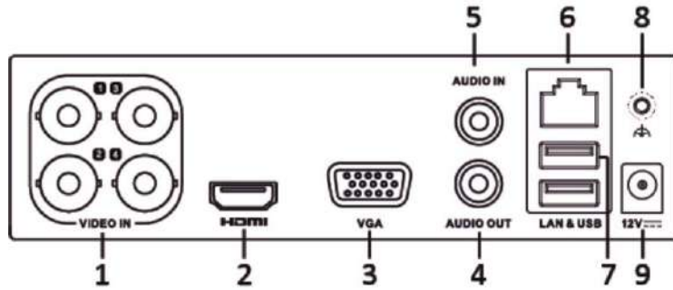
Рисунок 1-5 Задняя панель 1
