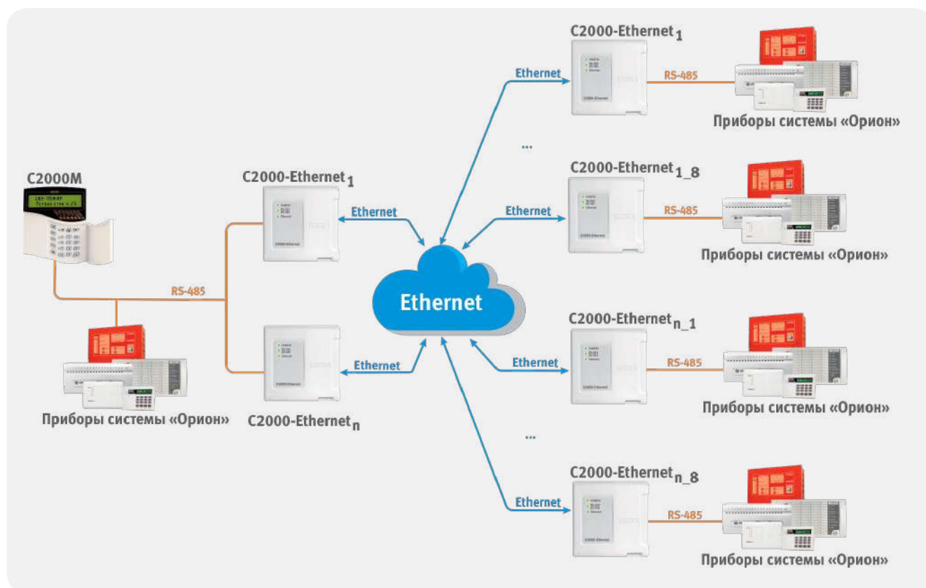
Рисунок 99. Структурная схема использования «С2000-Ethernet» с «С2000М»
