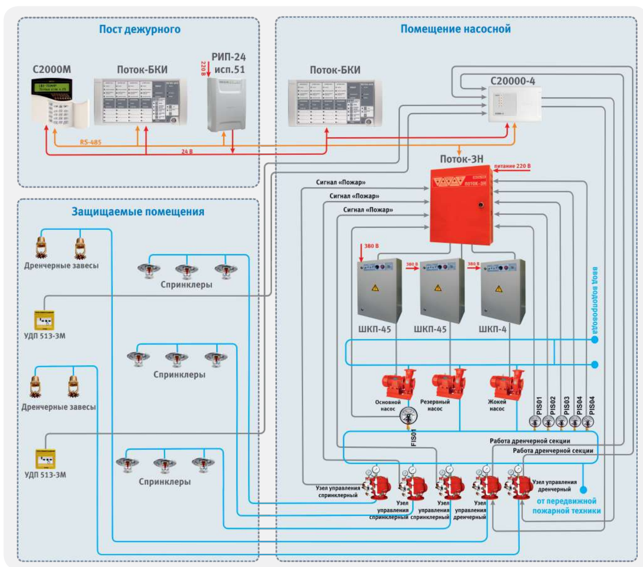
Рисунок 25. Автоматическая установка пожаротушения с тремя спринклерными и двумя дренчерными секциями
