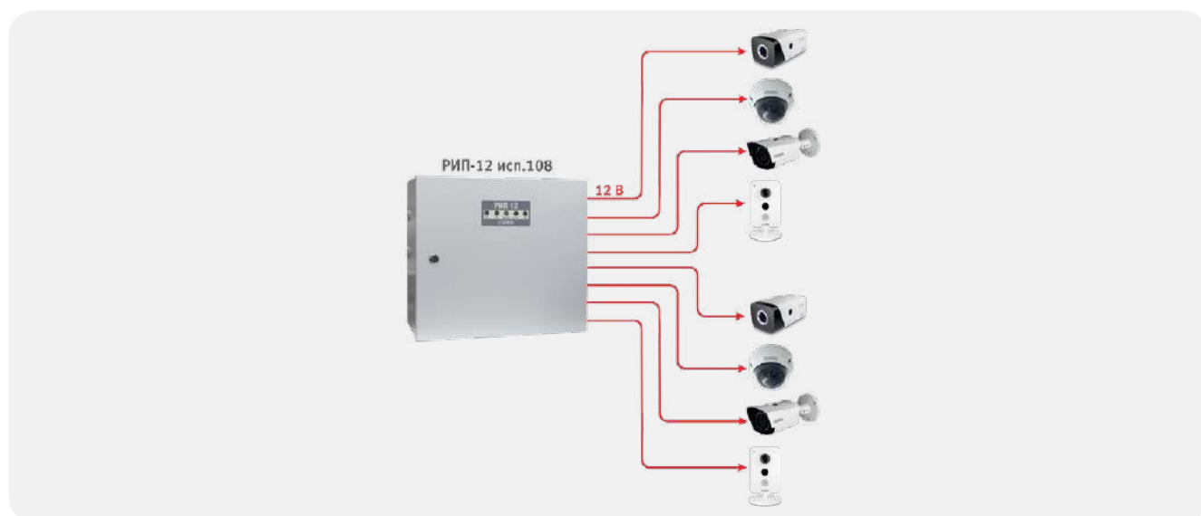
Рисунок 69. Организация питания видеокamер с помощью многоканального источника резервированного питания РИП-12 исп.108
