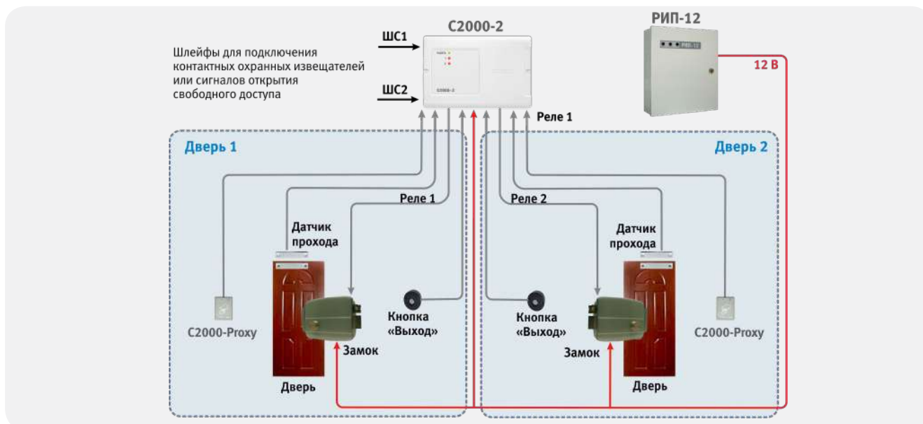
Рисунок 41. Режим работы «Две двери на вход»
