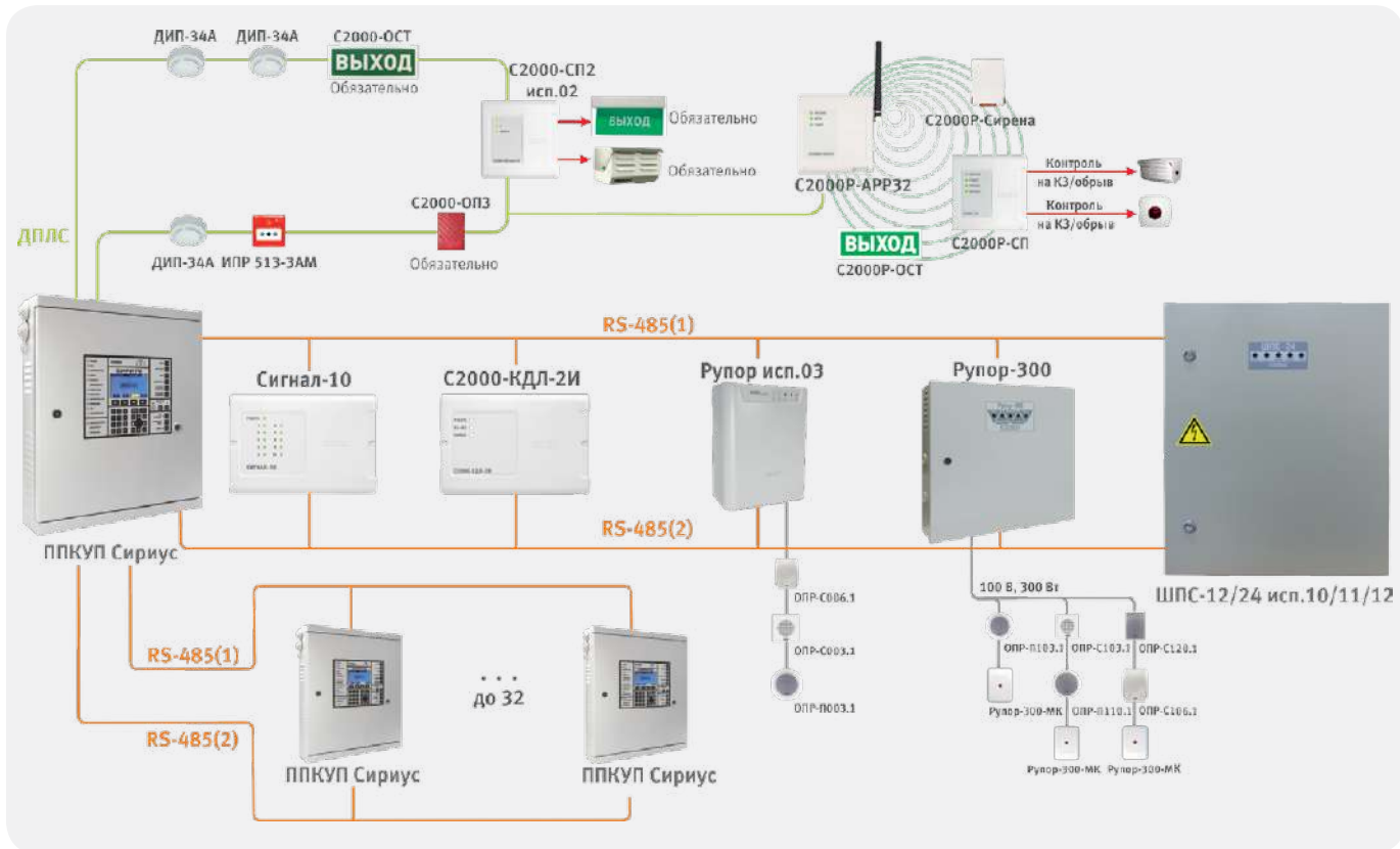
Рисунок 19. Система оповещения с повышенными требованиями к надежности
