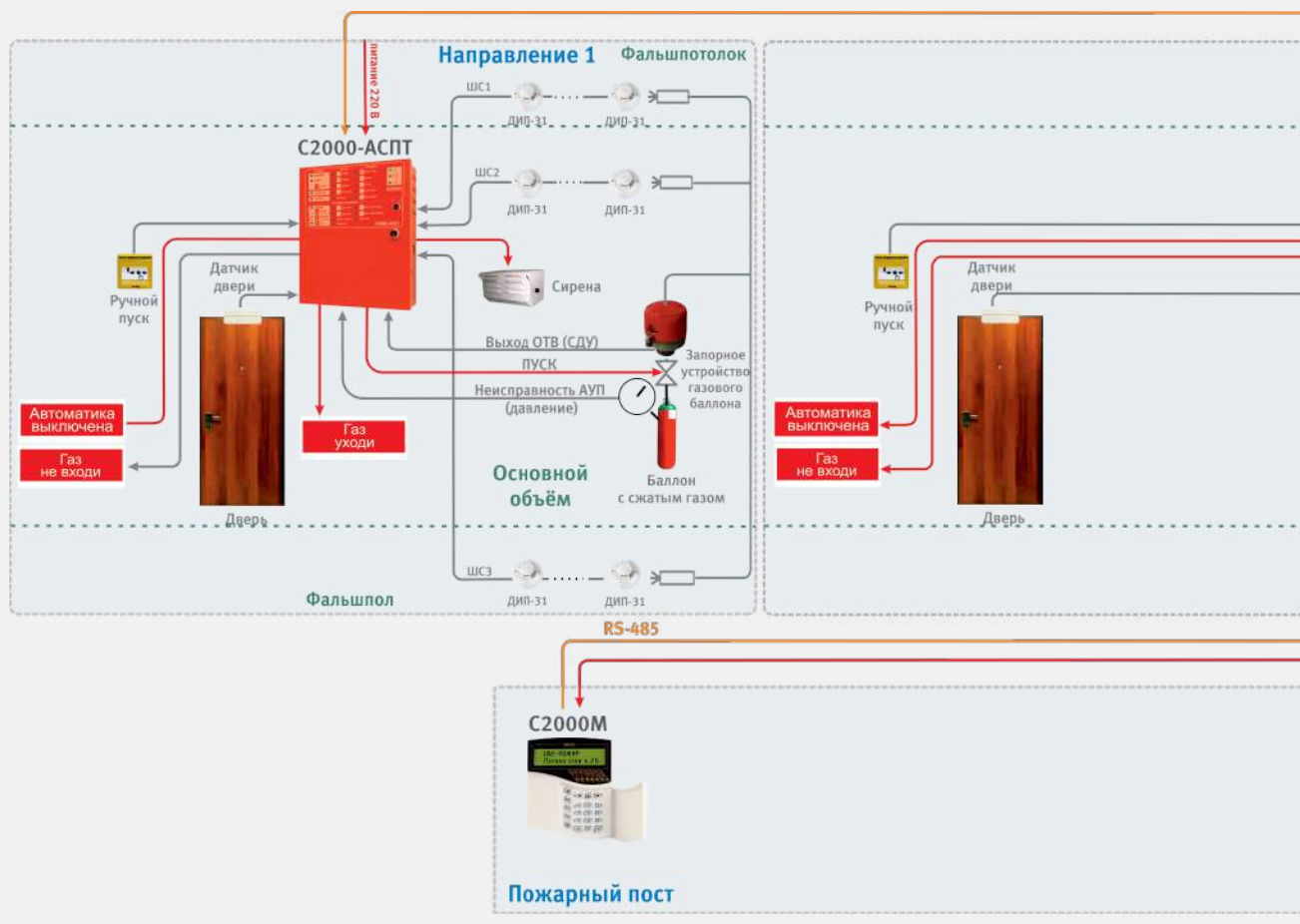
Рисунок 20. Распределенная установка газового пожаротушения
