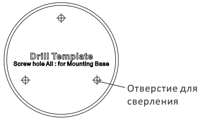
Рисунок 2-1 Шаблон крепления
